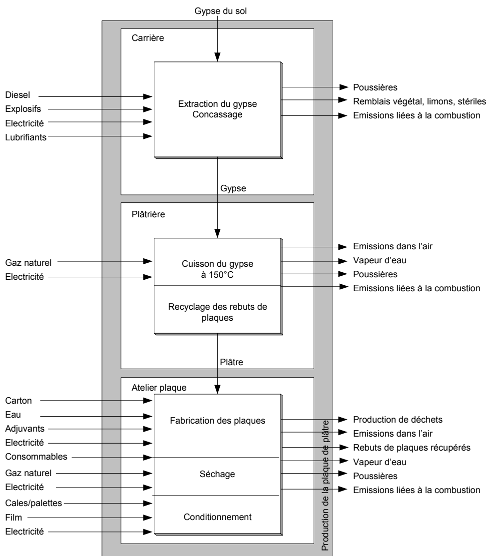
Figure 1 : Etapes de production des dalles de plâtre
